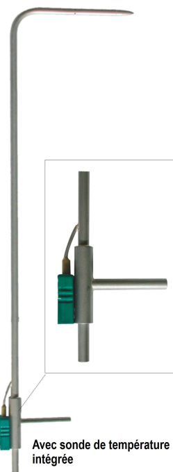
Tube de pitot type L avec TC K
